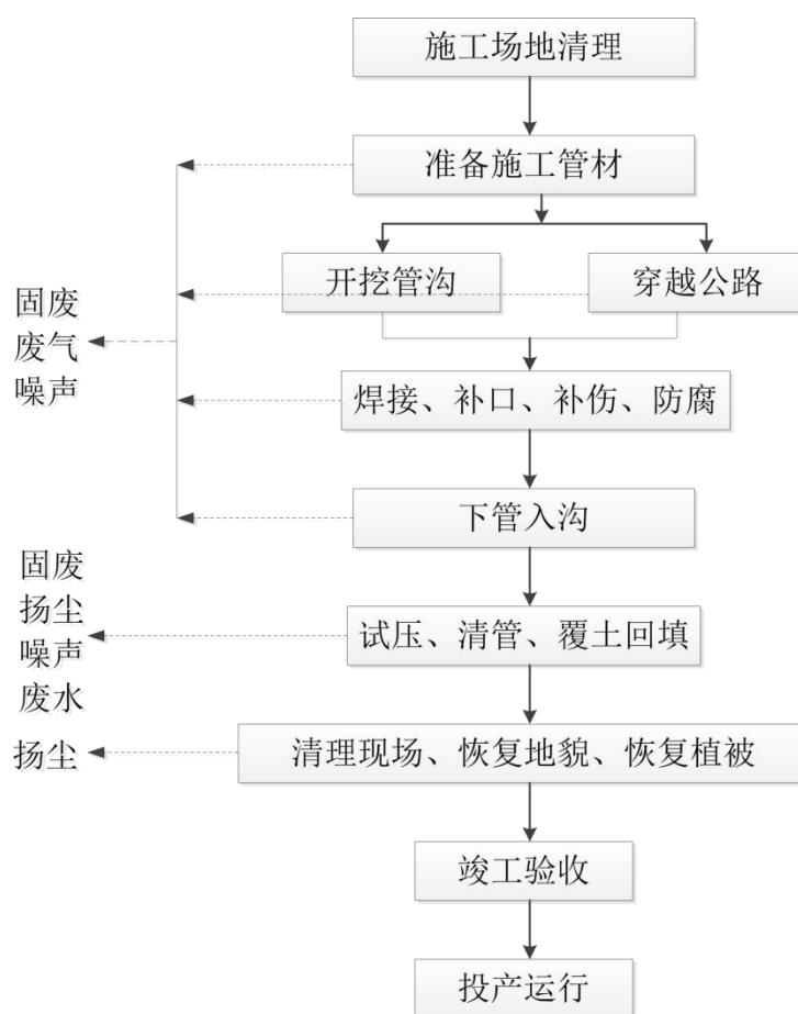
施工期管道施工工艺流程及产物示意图
