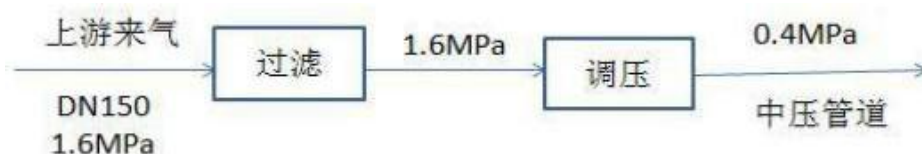
运营期管线工艺流程及产污节点图
